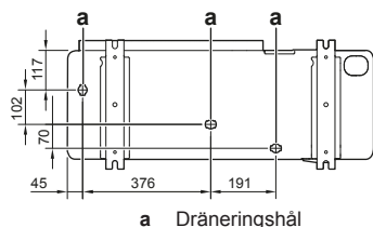
a Dräneringshål
