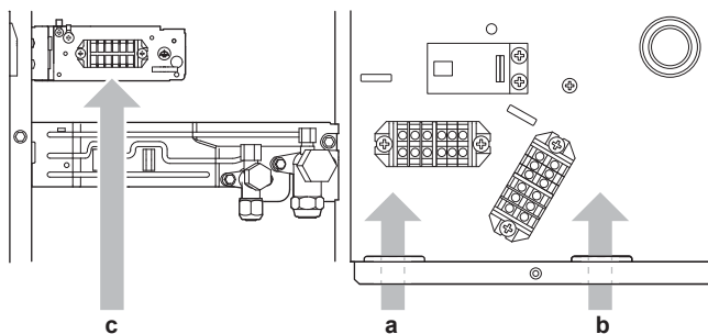
a Lågspänningskablar b Högspänningskablar c Nätspänningskabel
