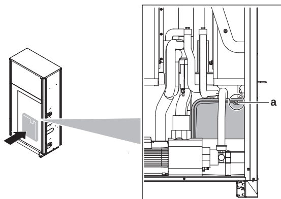
a Schraderventil
