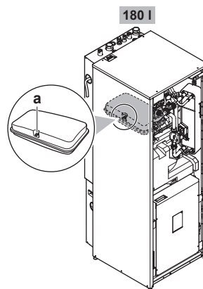
a Schraderventil
