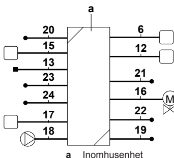
a Inomhusenhet
