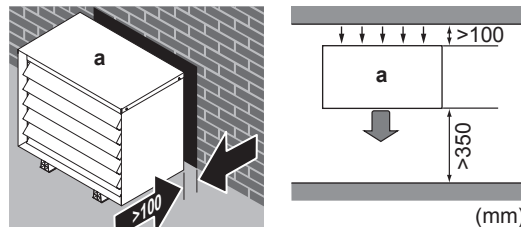
a Ljudskydd
