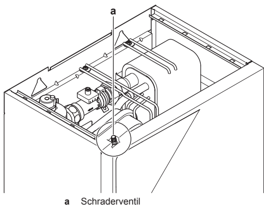
a Schraderventil
