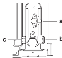
a Vätskestoppventil b Gasstoppventil c Serviceport
