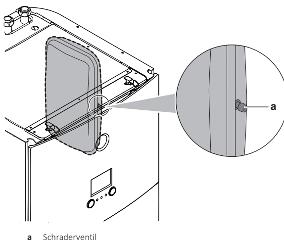
a Schraderventil
