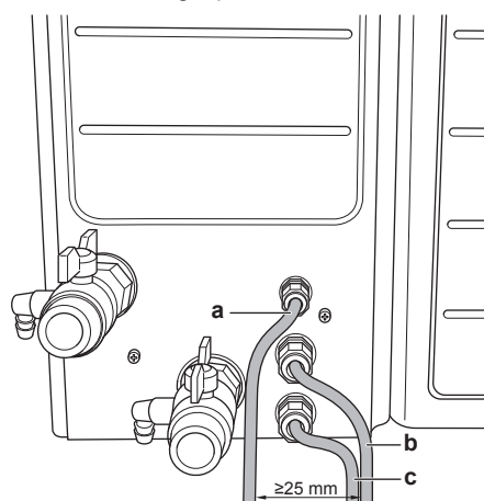
a Lågspänningskabel b Högspänningskabel c Nätspänningskabel
