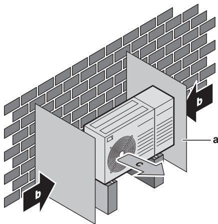
a Avskärningsplåt b Rådande vindriktning c Luftutlopp
