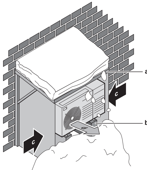
a Snöskydd eller skjul b Pelare c Rådande vindriktning d Luftutlopp
