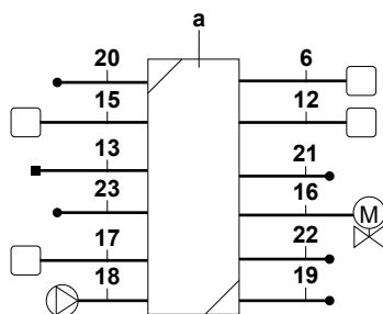
a Inomhusenhet
