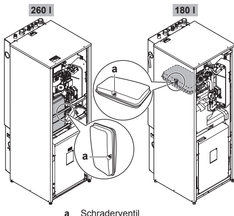
a Schraderventil
