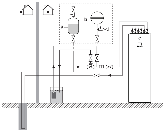
a Bärarnivåkärlet (tillbehör) b Expansionskärl (anskaffas lokalt, om det inte går att installera bärarnivåkärlet som högsta punkten)
