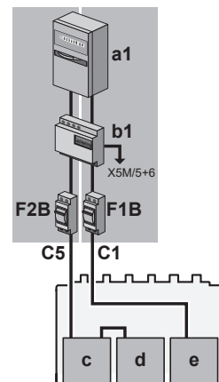
#2: Strömförsörjning med dubbel kabel (= delad strömförsörjning)
