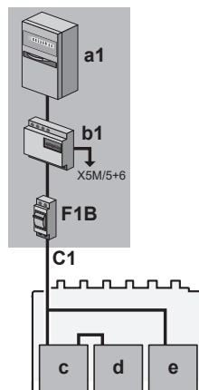
#1: Strömförsörjning med enkel kabel (= kombinerad strömförsörjning)
