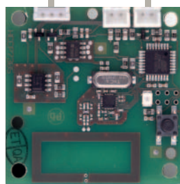
RF-MOTTAGARE
