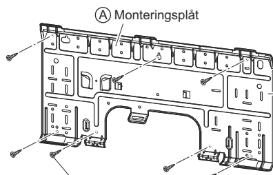
(B) Fästskruv för monteringsplåt (anskaffas lokalt: M4 x 25L)
