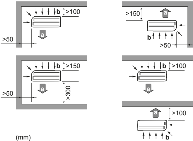
(mm) a Luftutlopp b Luftintag
