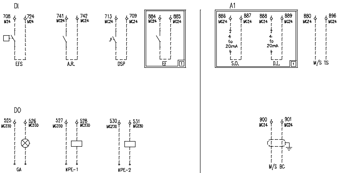
Figur 5 – Enhetens ledningsdragnig på installationsplatsen
