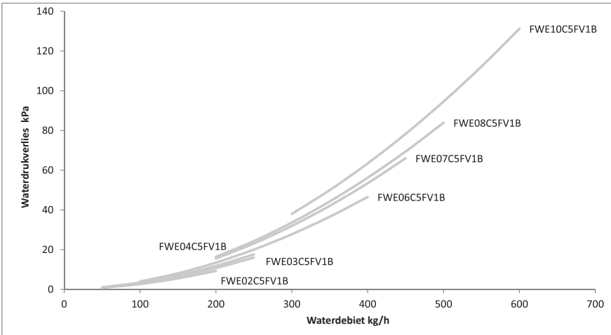
Waterdrukverlies 1-Rij Convector systeem
