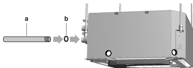
Fig. 4.9: Ansluta vattenledningarna
