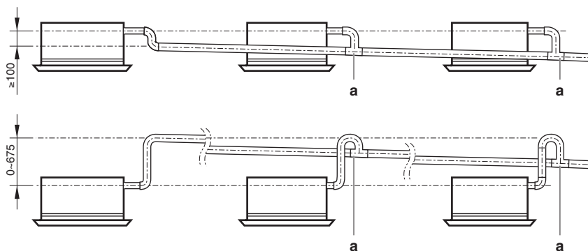
Fig. 4.18: Sammanföring av flera dräneringsledningar
