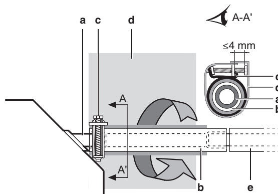
Fig. 4.20: Linda in tätningsdynan
