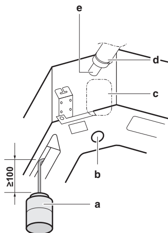
Fig. 4.21: Metod för tillsats av vatten
