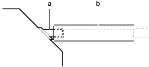
Fig. 4.19: Anslutning av dräneringsslangen
