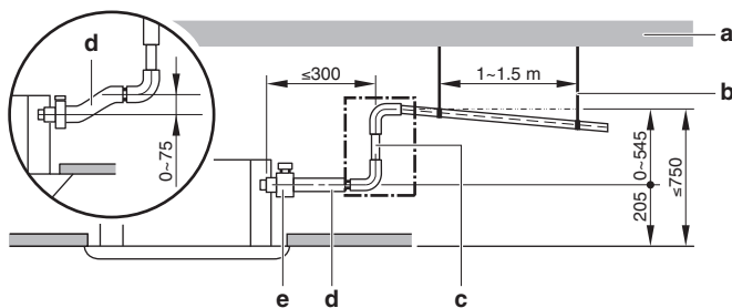
Fig. 4.17: Installation av dräneringsrör
