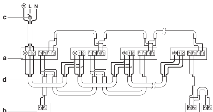
Fig. 4.14: Gruppkontroll eller användning av 2 fjärrkontroller
