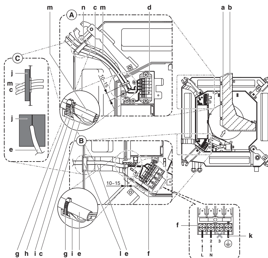
Fig. 4.15: Anslutning av elledningarna
