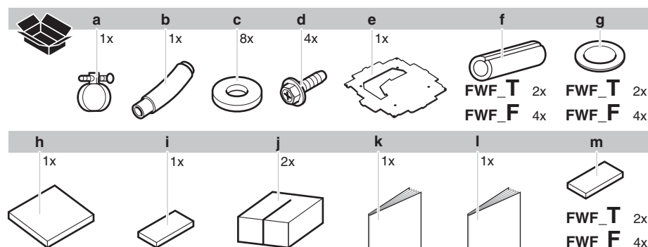
Fig. 4.1: Tillbehör
