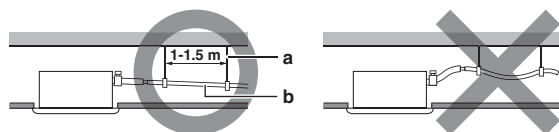
Fig. 4.16: Installation av dräneringsrör
