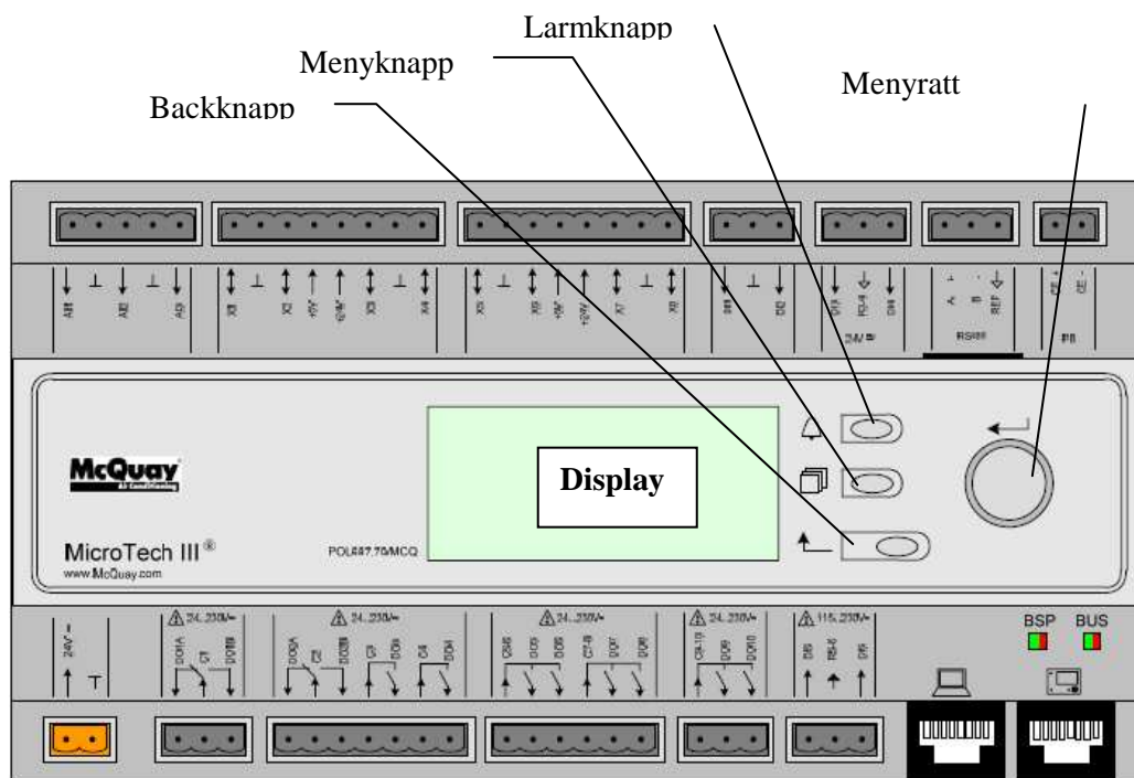
Fig. 7 - Styrsystem
