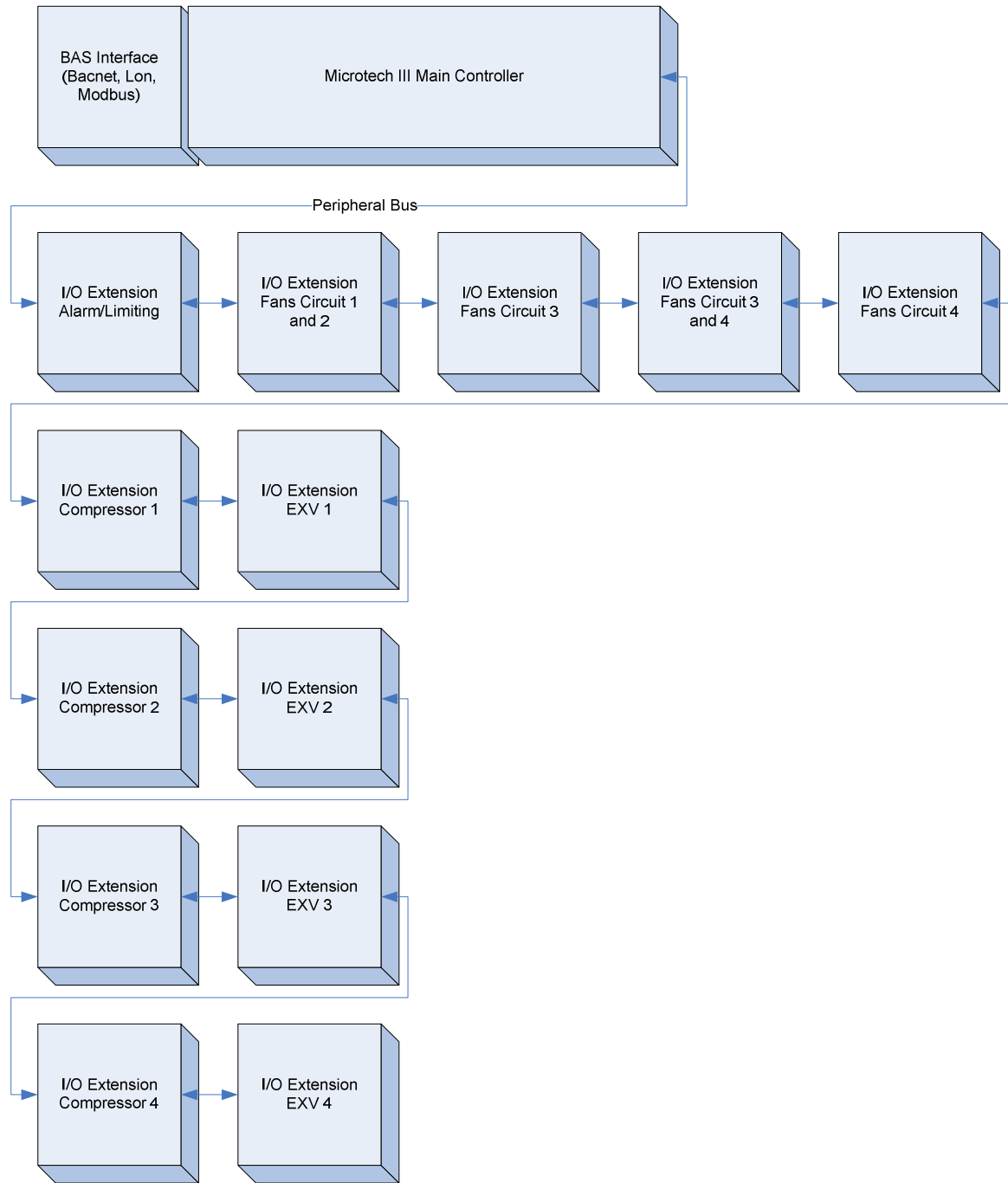
Fig. 4 - Systemuppbyggnad
