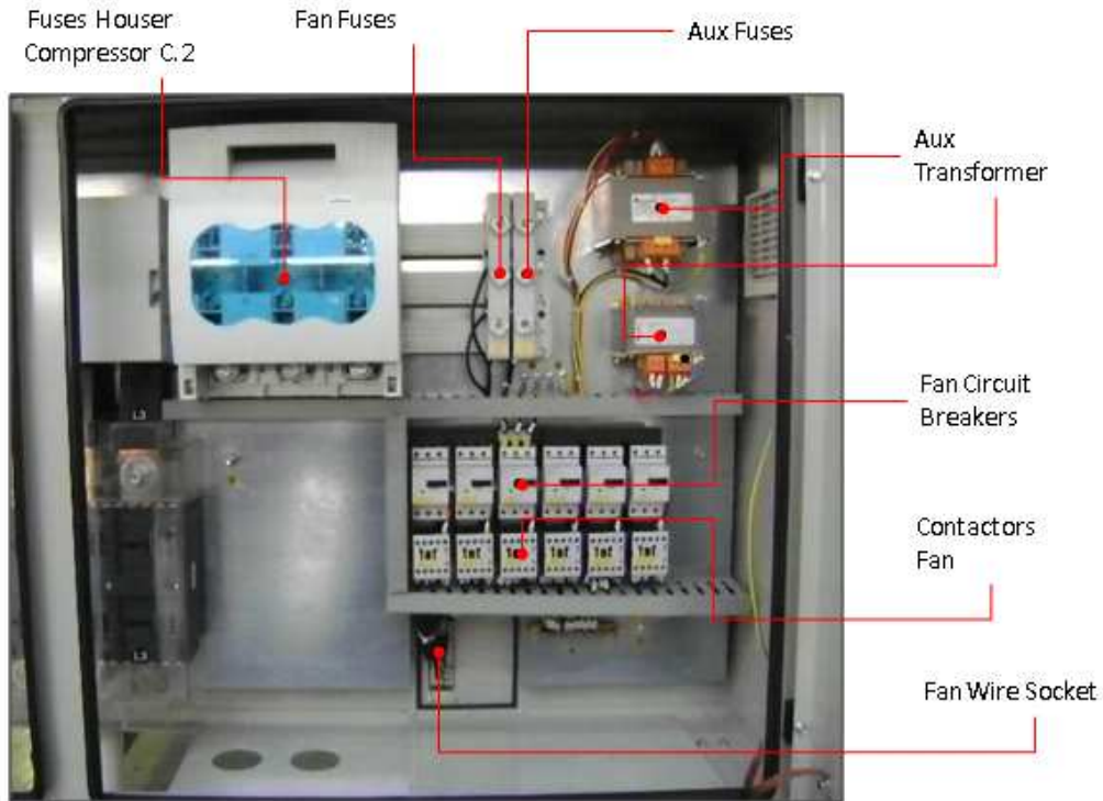
Fig. 3 - Eltavla, höger sida
