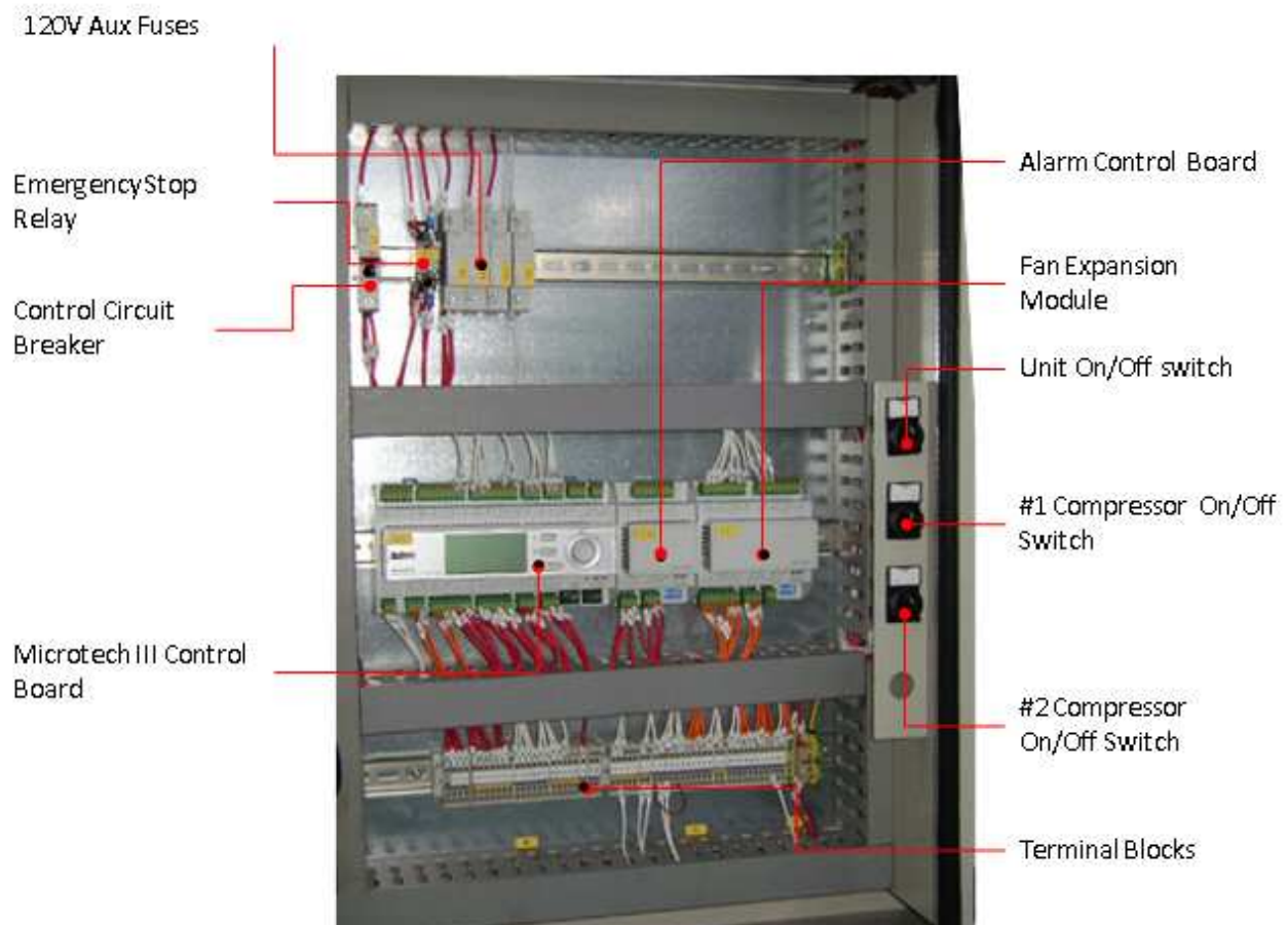
Fig. 1 - Manöverpanelens delar
