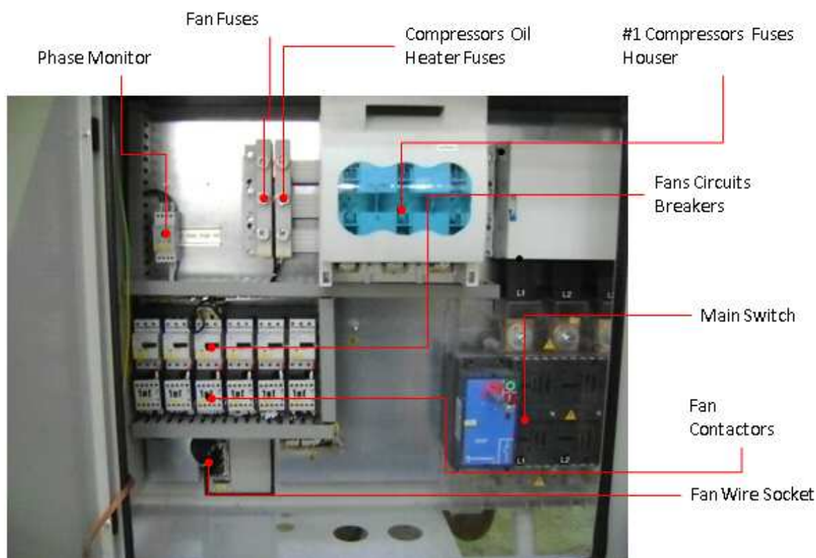
Fig. 2 - Eltavla, vänster sida
