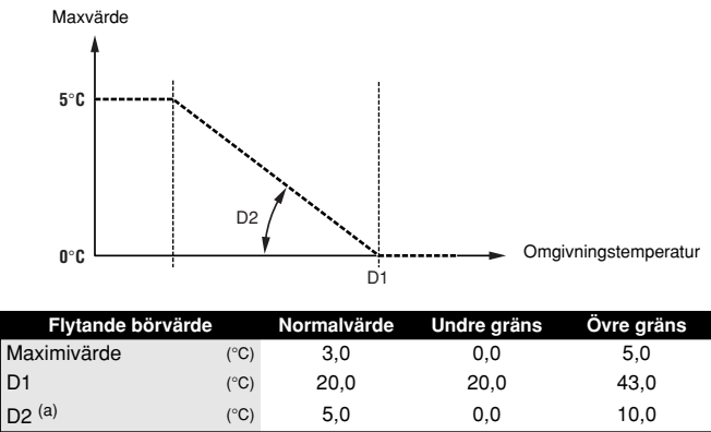
(a) ökningen av flytande börvärde för 10°C fall av omgivningstemperaturen
